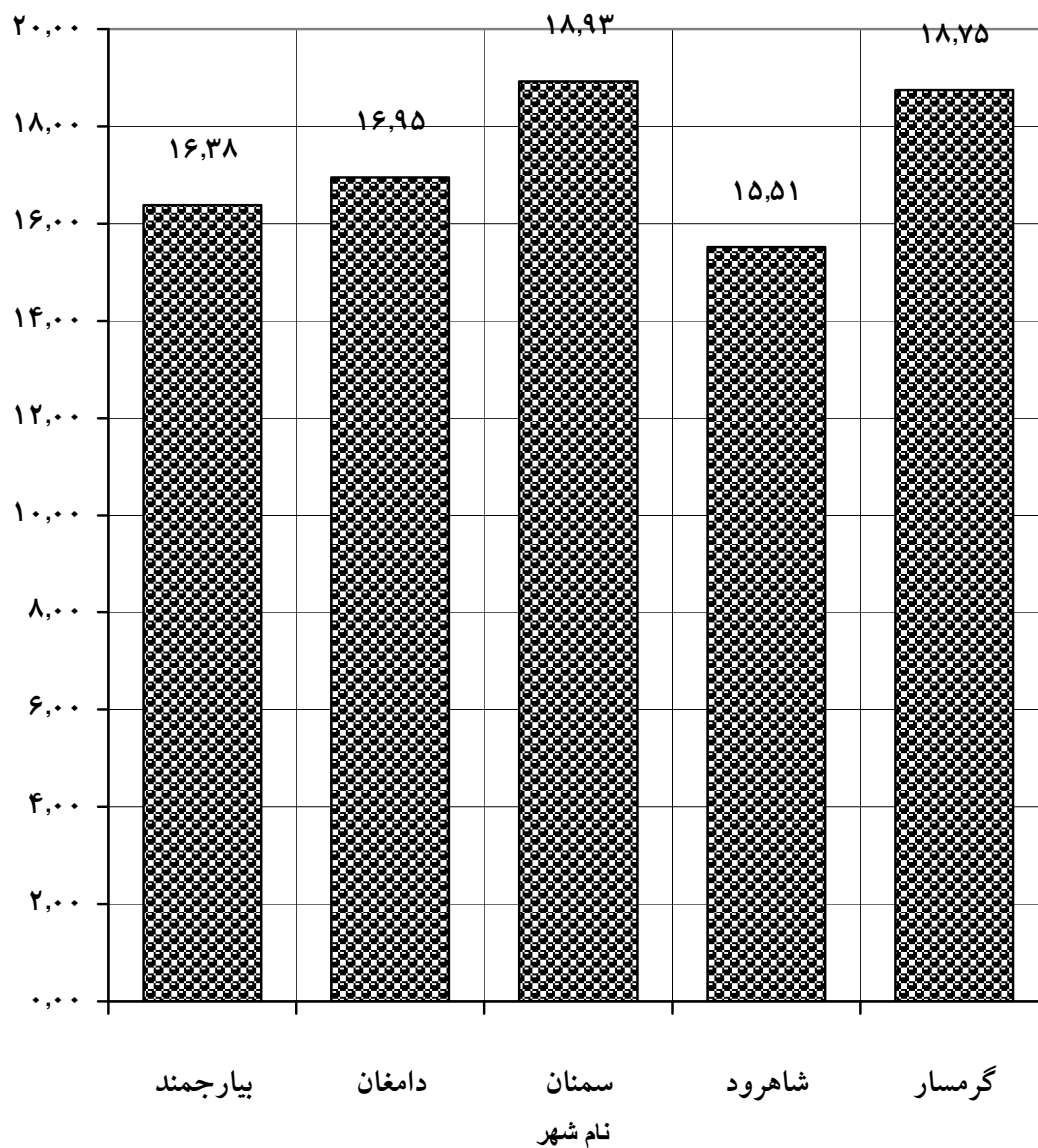
نمودار متوسط دمای هوای شهرهای دارای ایستگاه سینوپتیک استان سمنان: ۱۳۸۸ سانتی گراد
